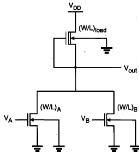
FIG.CIRCUITDIAGRAMOFNORGATE
