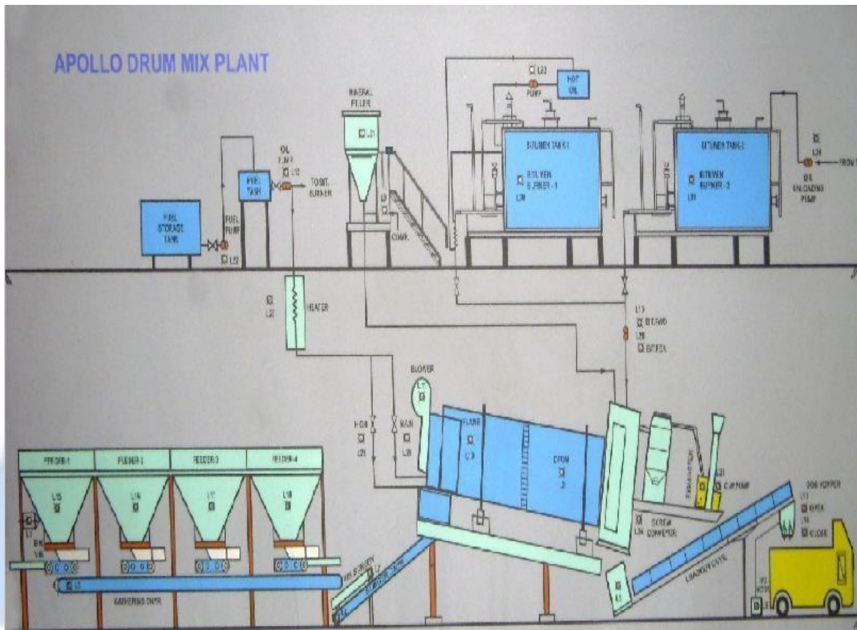
Fig.SchematicDiagramofDrumMixPlant
