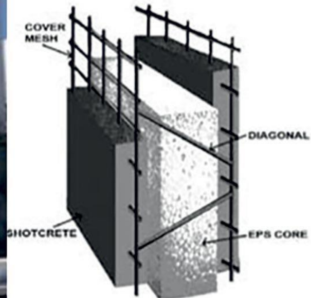
Figure6:ExpandedPolystyrene(EPS)corepanelsystem
