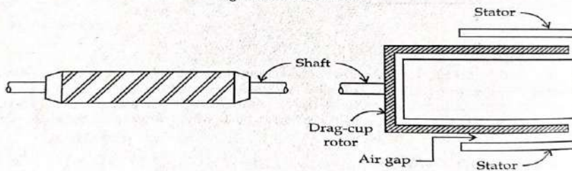
Fig. 9.4. a.c. servomotor
