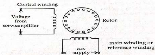
Fig. 9.4. a.c. servomotor
