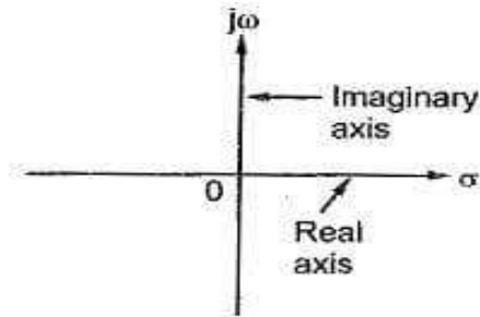
(a) s-plane
